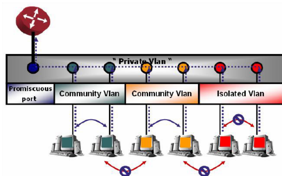
(그림) 사설 VLAN 개념도
