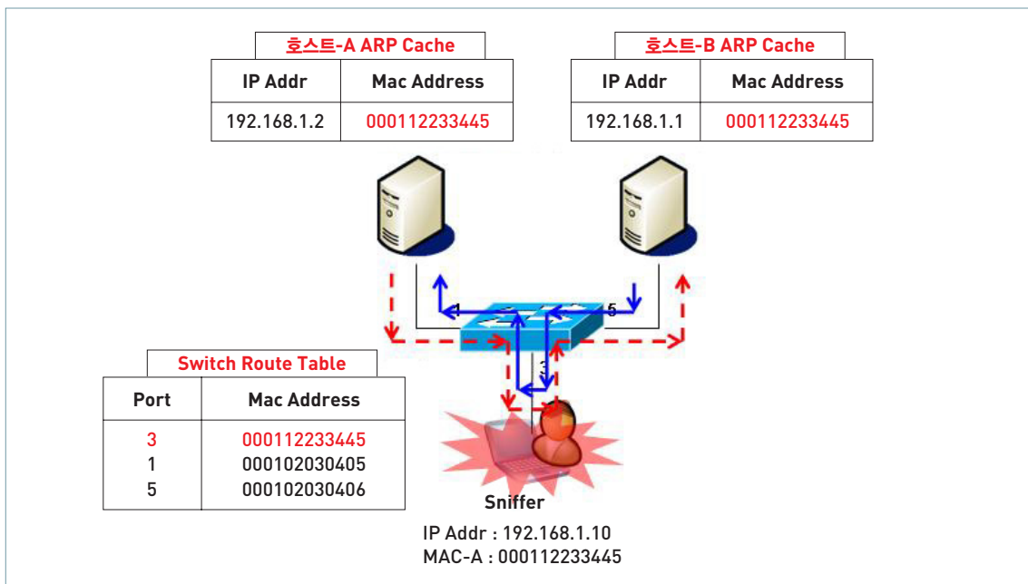
(그림) ARP Spoofing후 스니핑
