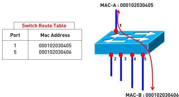
(그림) 두 호스트 간 스위치 통신
